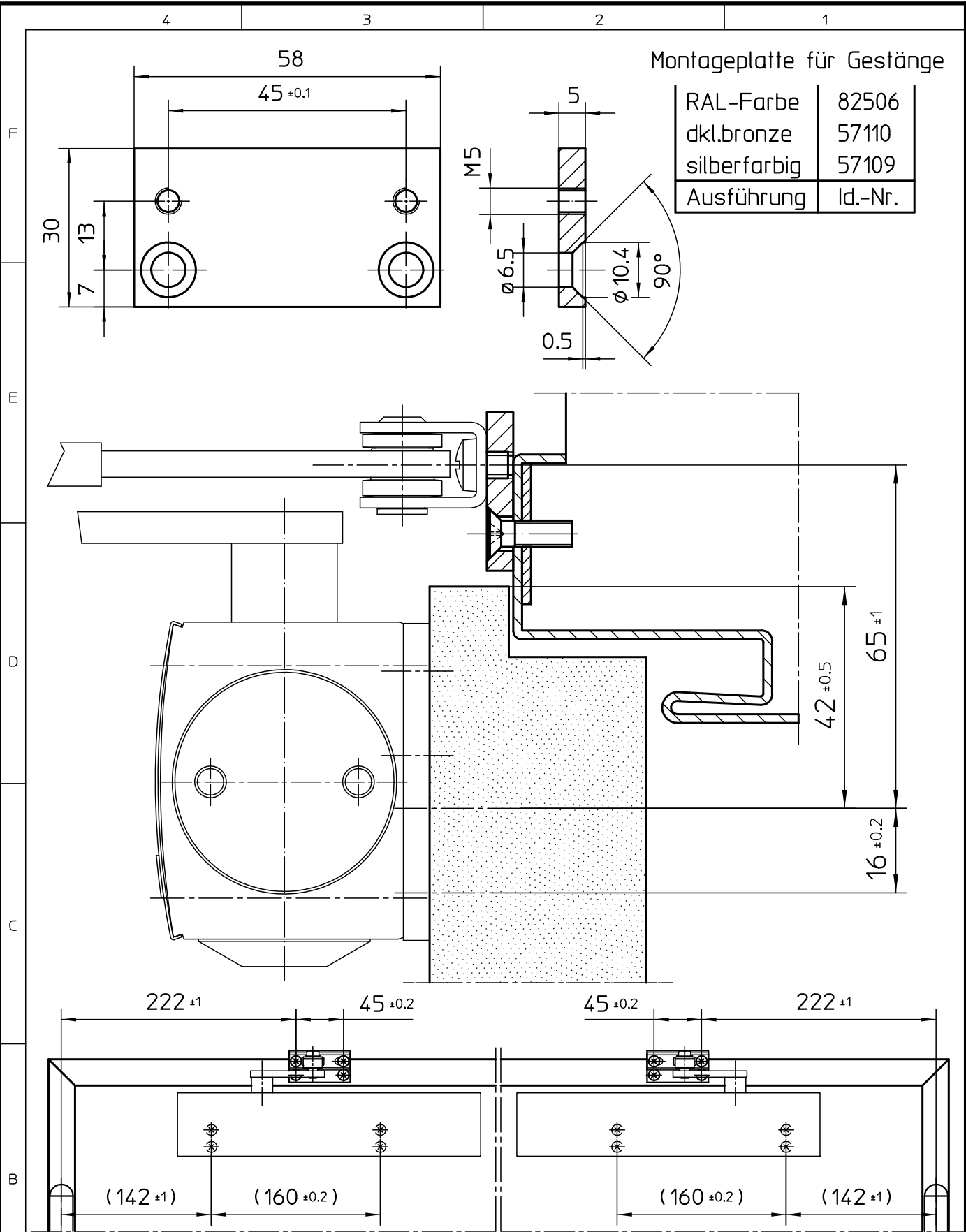
Anschlagmaße für Tür mit Linksflügel
