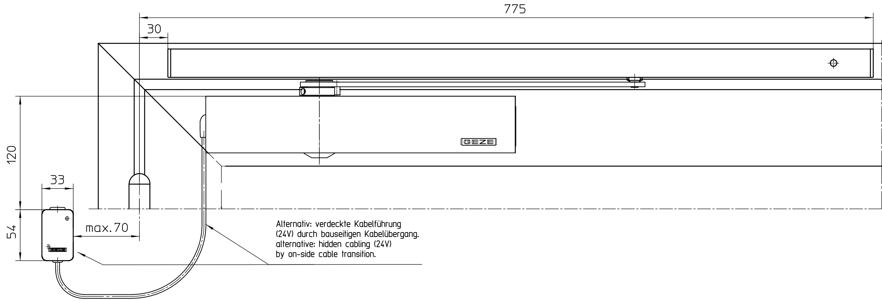
Direktbefestigung/Direct mounting
