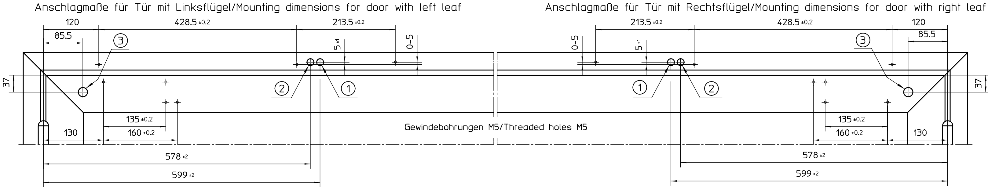
Direktbefestigung/Direct mounting
