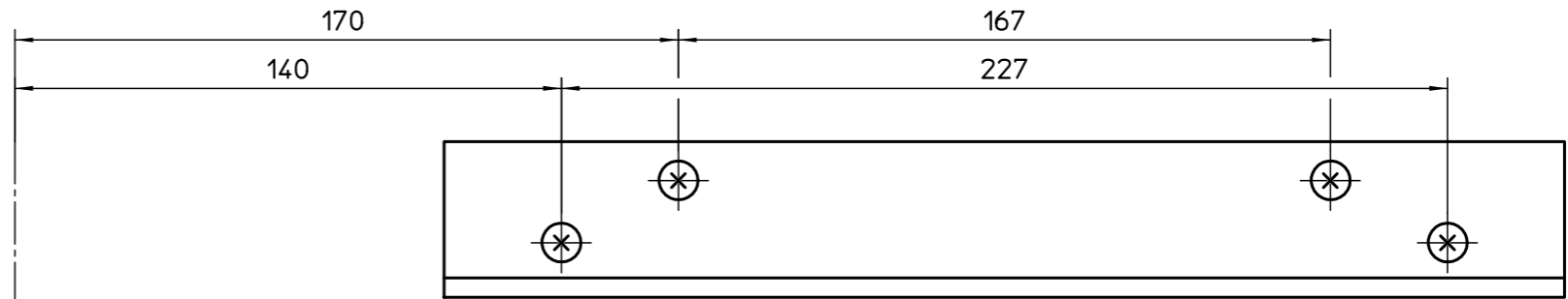
Ansicht X ohne Schließer und Türblatt gezeichnet
