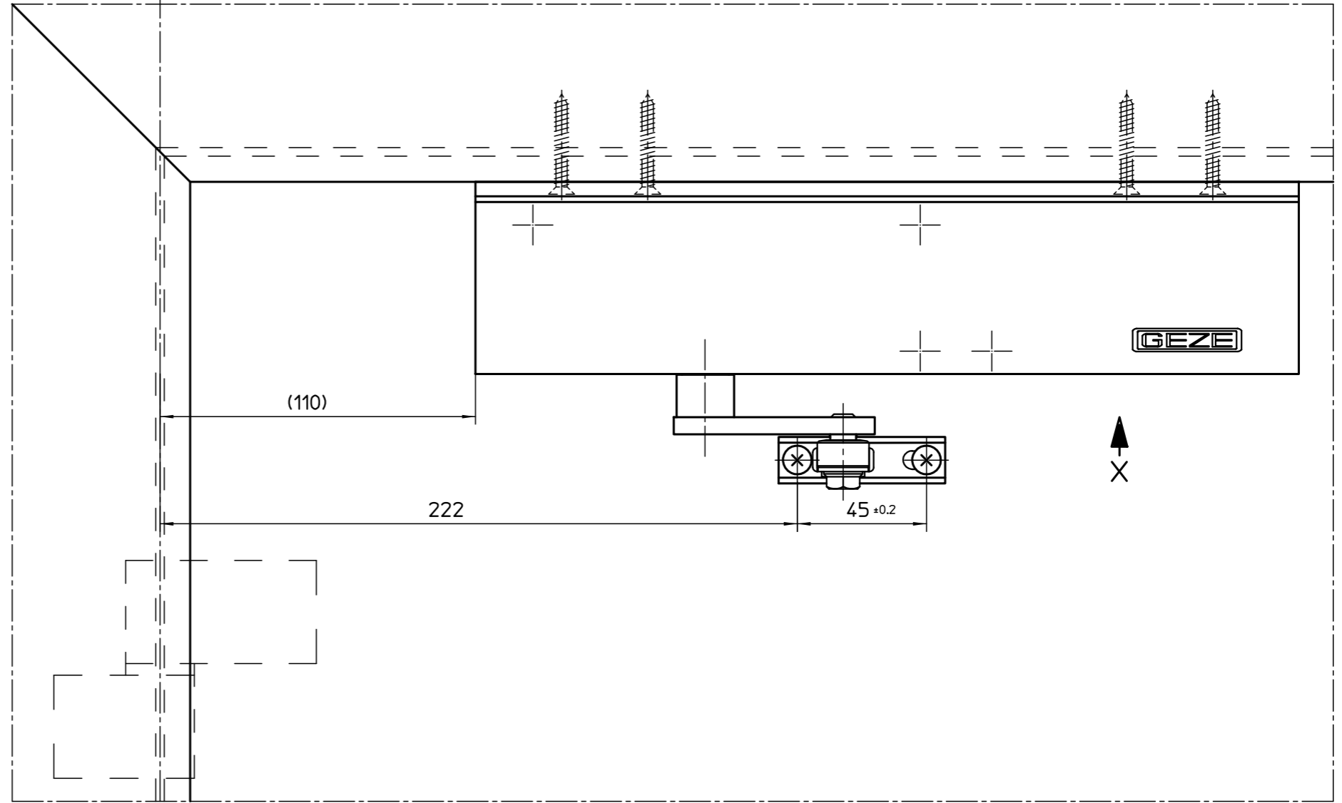
Ansicht X ohne Schließer und Türblatt gezeichnet
